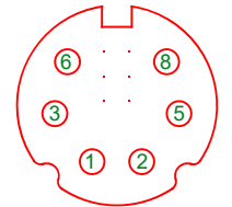
6 WAY DIN PIN VIEW
