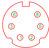
6W MINI DIN PIN VIEW
